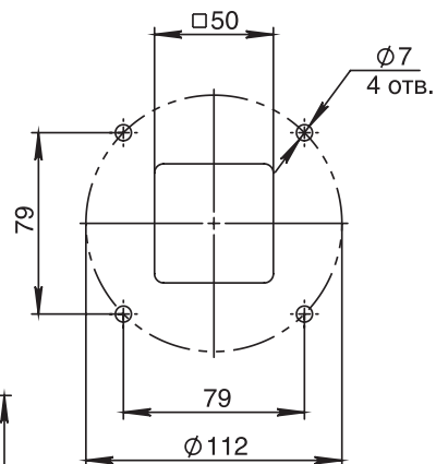
монтажный вырез
