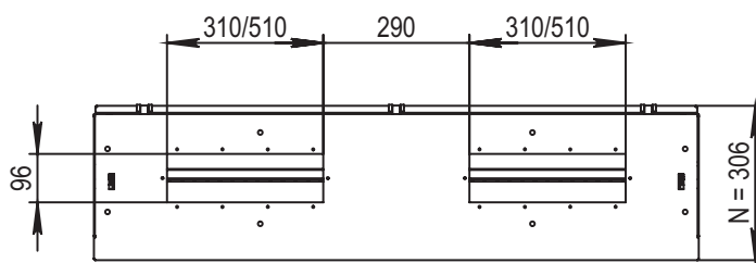
Вид снизу
