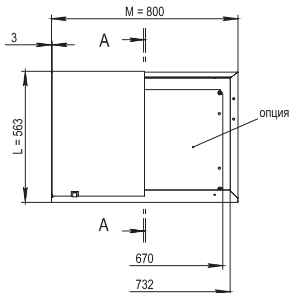
Вид снизу
