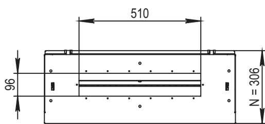
Вид снизу
